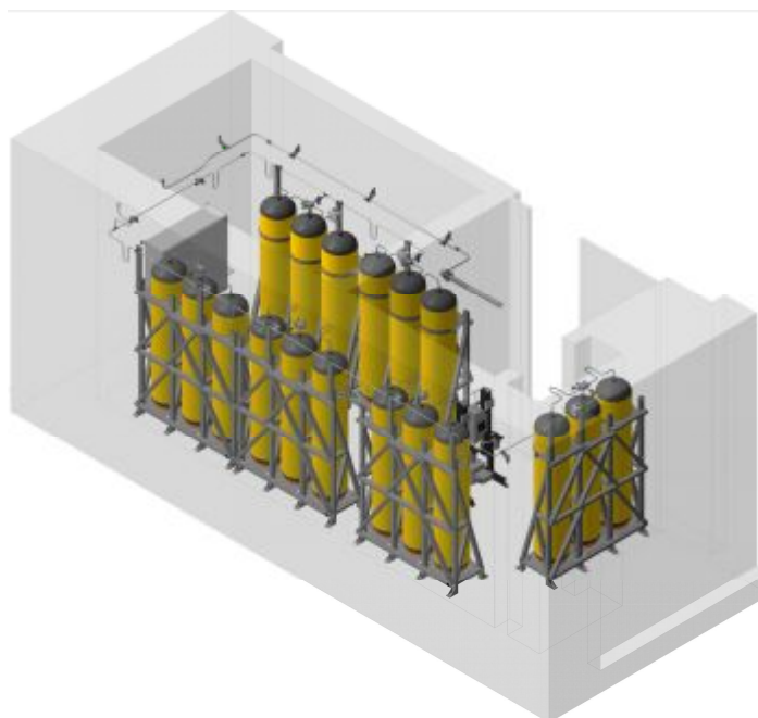
Типовая компоновка БСЖО в помещении АЭС
